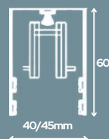
PLISSÉE LATÉRALE (Coupe verticale)
