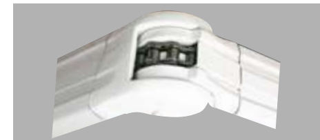
Bras testés à 60 000 cycles dotés d'une articulation chaîne à rouleaux.
